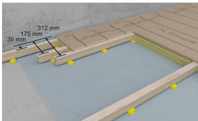
Figur 4 Klimagulv med kantstrø 35 mm c-c fra væg og med ekstra strø under vendespor og under samling mellem vendeplader og gulvplader, se monteringsanvisningen for Kronospan vendeplader.
