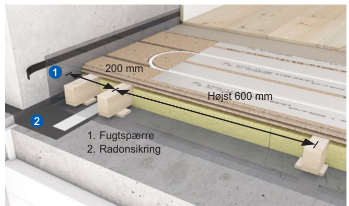
Figur 2 Klimagulv lagt på strøer med fræsedede vendespor udført på byggepladsen.
