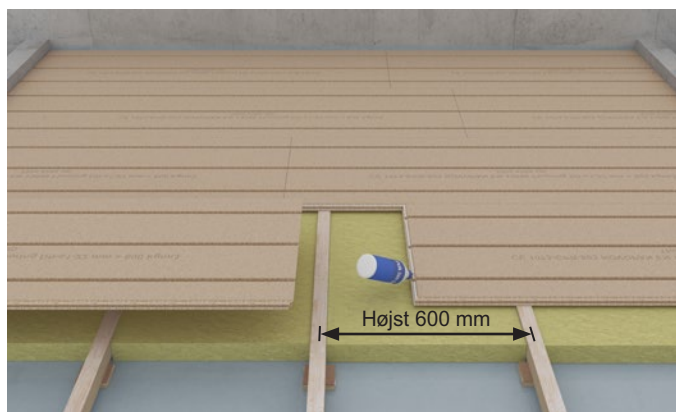
Figur 5 Klimagulv lagt i forbandt med flyvestød og pladeforskydning på mindst 300 mm. Må kun anvendes i almindelige boligrum.
